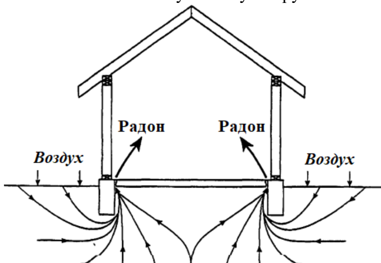
Рисунок 1 – Поступление радона в частное домостроение с фундаментной плитой на грунтовом основании
