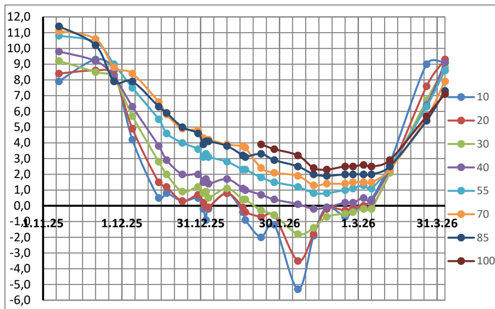
Рисунок 2 – Динамика температуры почвы на разной глубине осенью, зимой и весной 2025–2026 гг.
