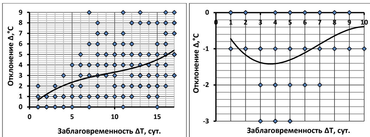
Рисунок 2 – Зависимость ошибки прогноза от заблаговременности в 2025 г.
