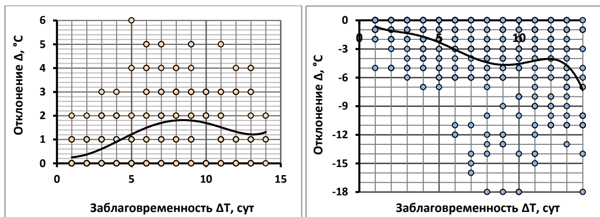
Рисунок 3 – Зависимость ошибки прогноза от заблаговременности в 2026 г.
