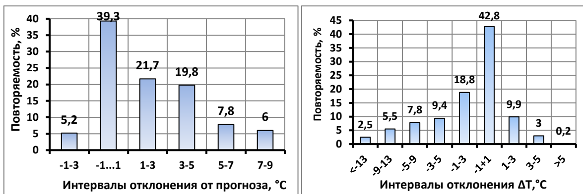
Рисунок 1 – Распределение повторяемости отклонений прогнозной температуры от фактической по интервалам их варьирования
