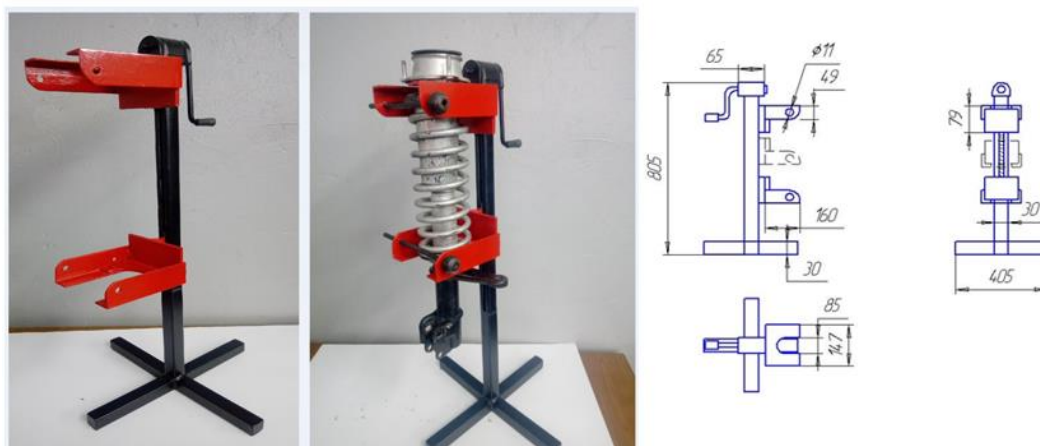
Рисунок 2 – Стенд для стяжки пружин подвески легковых автомобилей
