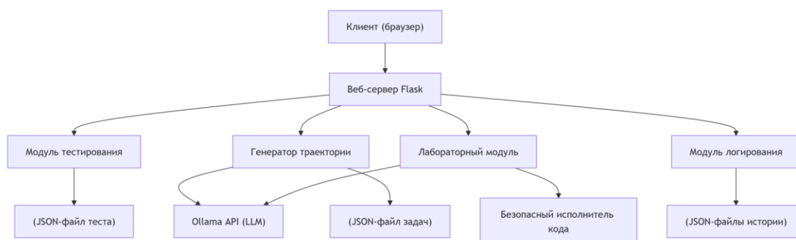
Рисунок 1 – Общая архитектура системы
