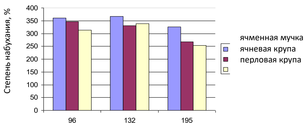
Рисунок 3 – Влияние степени измельчения на процесс набухания
