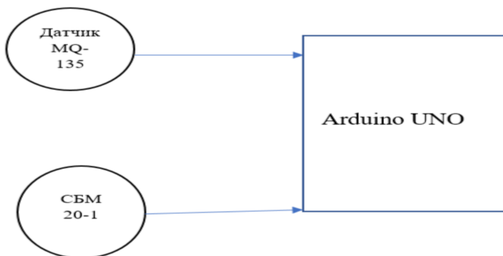
Рисунок 1 – Блок-схема детектора.
