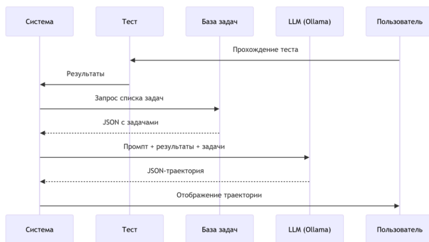
Рисунок 2 – Процесс генерации индивидуальной траектории
