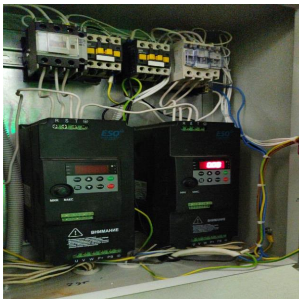
Рисунок 1 – Частотники серии ESQ-230
