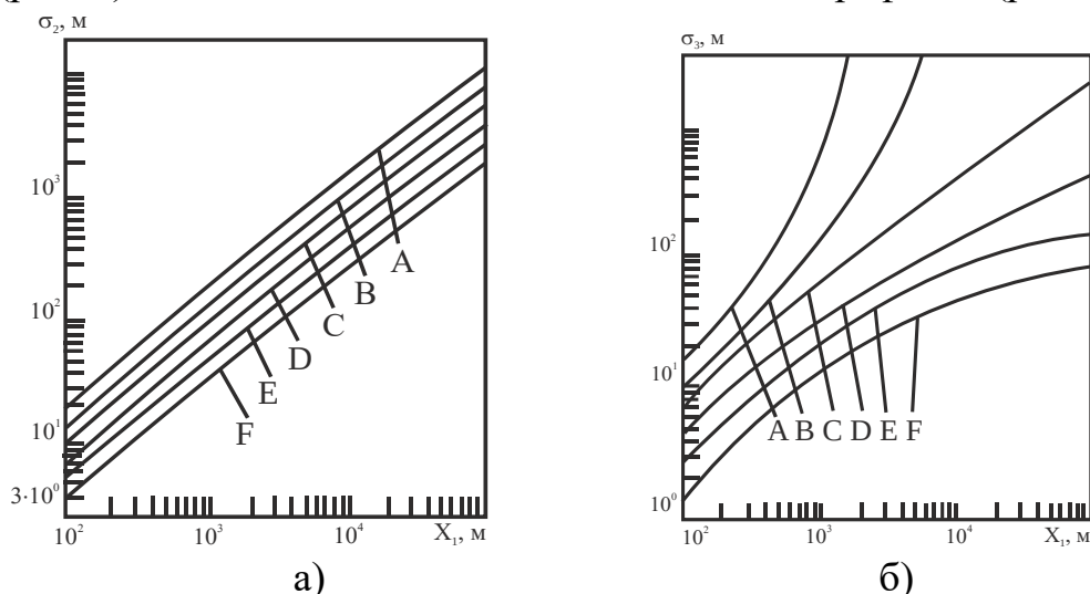
Рисунок 2 – Стандартные отклонения в зависимости от расстояния к источнику и категории стойкости погоды: а – для поперечного и горизонтального; б – для вертикального распределения концентраций.
