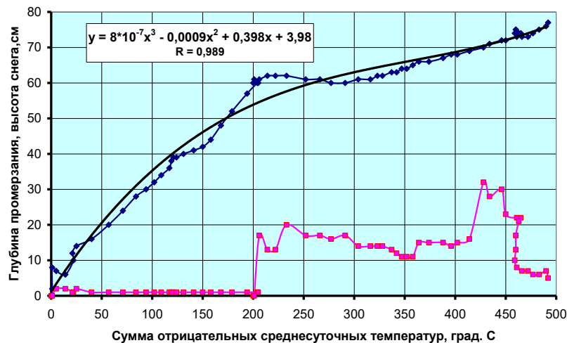
Рисунок 1 – Нарастание глубины промерзания почвы (верхняя линия) в зависимости от суммы отрицательных температур и высоты снежного покрова (нижняя линия)
