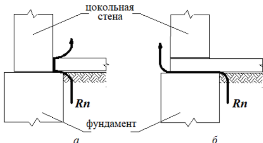
Рисунок 2 – Сопряжение фундаментной плиты с цокольной стеной: а – нерациональное; б – рациональное [5]
