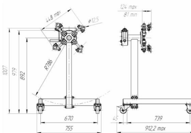
Рисунок 4 – Кантователь для разборки/сборки двигателей автомобилей
