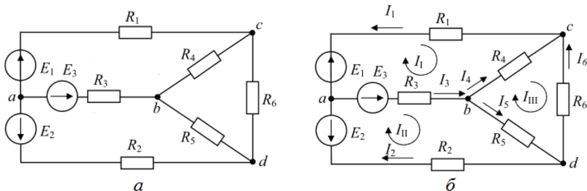
Рисунок 1 – Расчет электрической цепи по законам Кирхгофа: а – исходное задание; б – процедура решения
