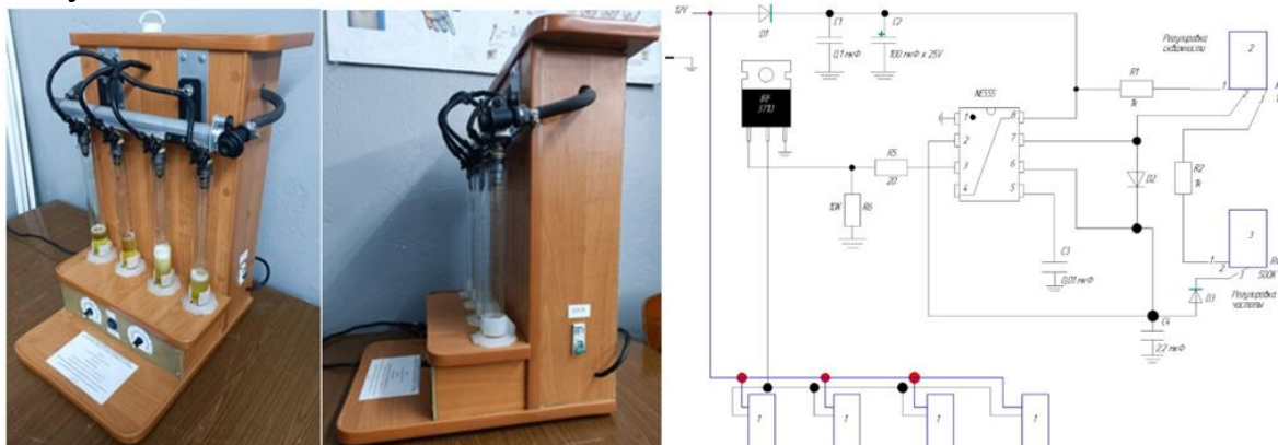
Рисунок 1 – Стенд для промывки и диагностики форсунок бензиновых двигателей
